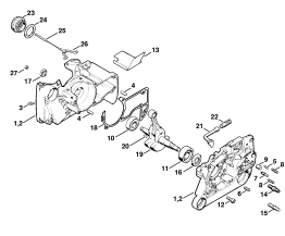
Kliková skříň
