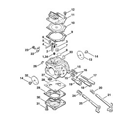
Karburač WJ-67
