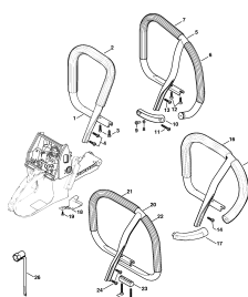
Trubka rukojeti
