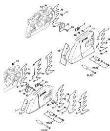
Viko řetězky
