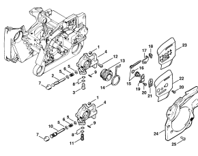
Olejové čerpadlo, zařízení pro napínání řetězu
