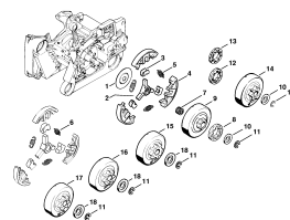
Spojka, řetězka
